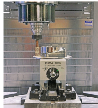
Fraisage de pièces complexes.
